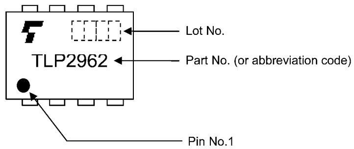
图 14.1 現品表示
