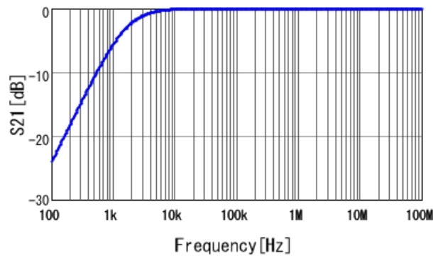
Sパラメータ S21
