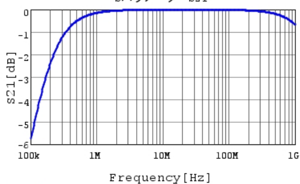
sパラメータ S21
