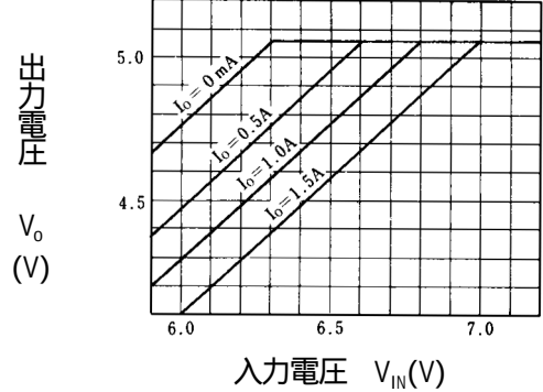
NJM7812 入出力間電位差特性例 ( T_j = 25 )
