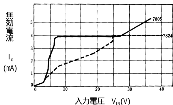
NJM7805/24 無効電流特性例 ( T_j = 25 )
