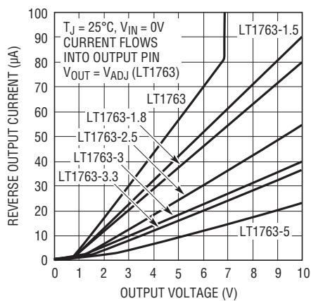
逆出力電流
