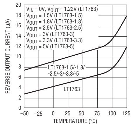
逆出力電流
