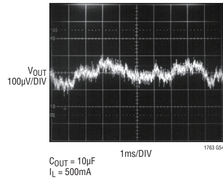
LT1763-5の 10Hz~100kHz出力ノイズ C_{BYP} = 1000\text{pF}
