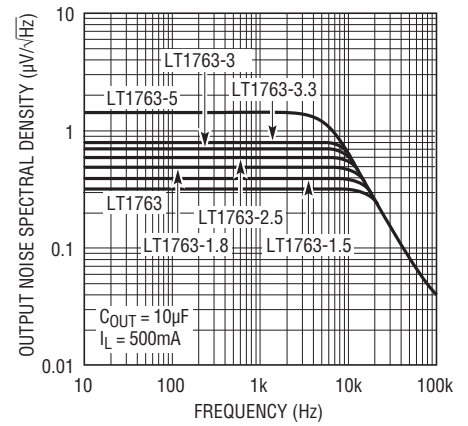
出力ノイズのスペクトル密度 C_{BYP} = 0
