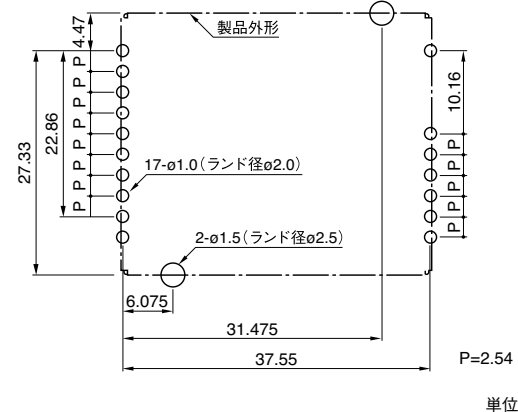
推奨基板取付け寸法
