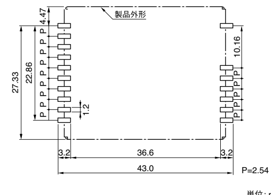
推奨基板取付け寸法
