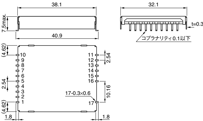
形状・寸法
