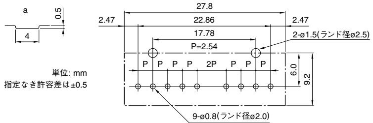
推奨基板取付け寸法
