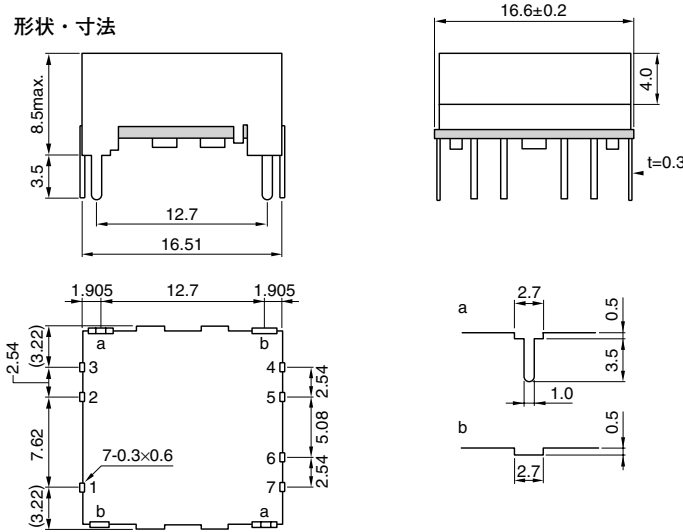
形状・寸法
