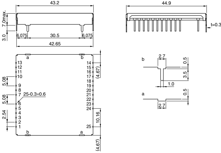
形状・寸法
