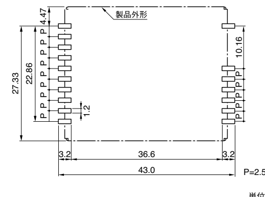
推奨基板取付け寸法
