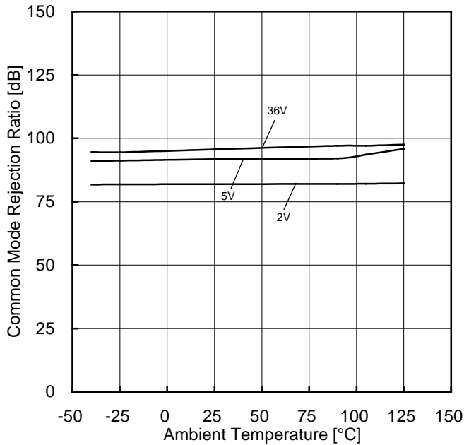
Figure 104. 同相信号除去比-温度特性
