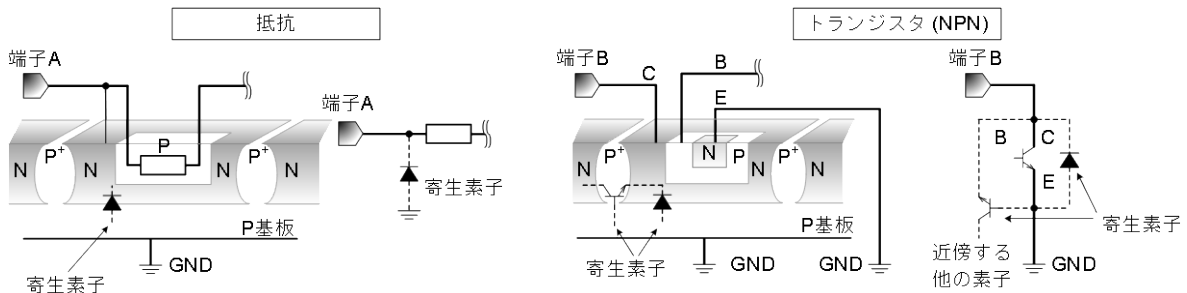
Figure 116. モノリシック IC 構造例
