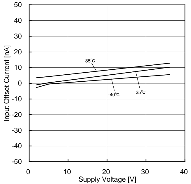
Figure 56. 入力オフセット電流-電源電圧特性
