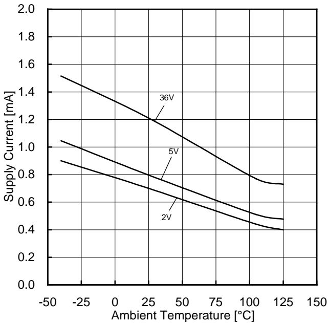
Figure 90. 回路電流-温度特性
