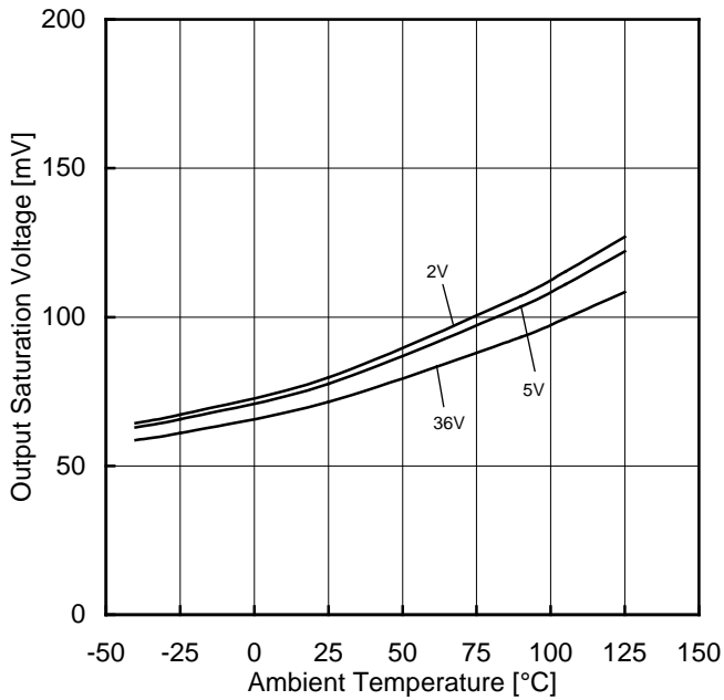
Figure 92. 出力飽和電圧-温度特性 ( I_{SINK}=4mA )
