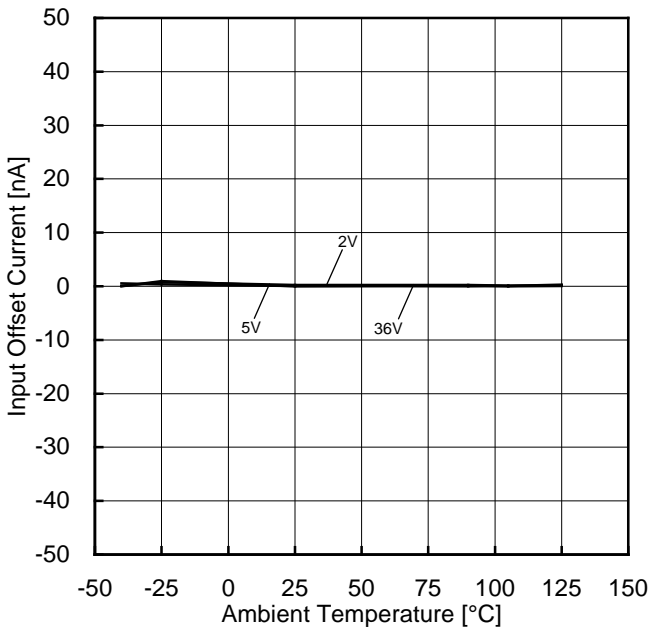
Figure 100. 入力オフセット電流-温度特性
