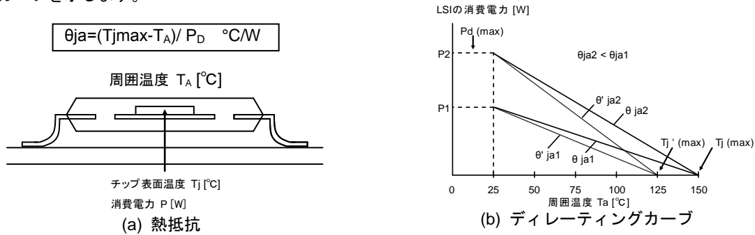
Figure 114. 熱抵抗とディレーティングカーブ
