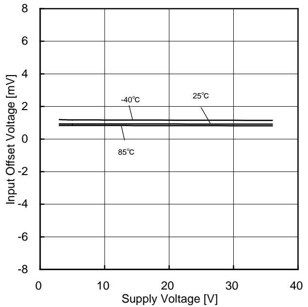
Figure 9. 入力オフセット電圧-電源電圧特性
