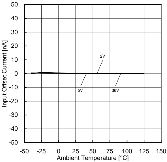
Figure 77. 入力オフセット電流-温度特性
