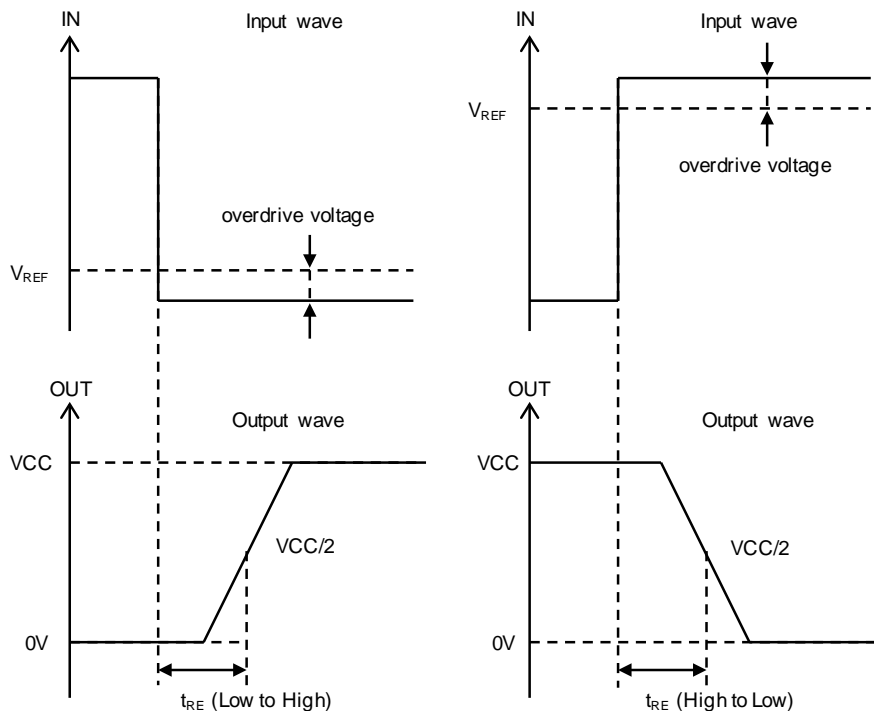
Figure 113. 応答時間測定時 入出力波形
