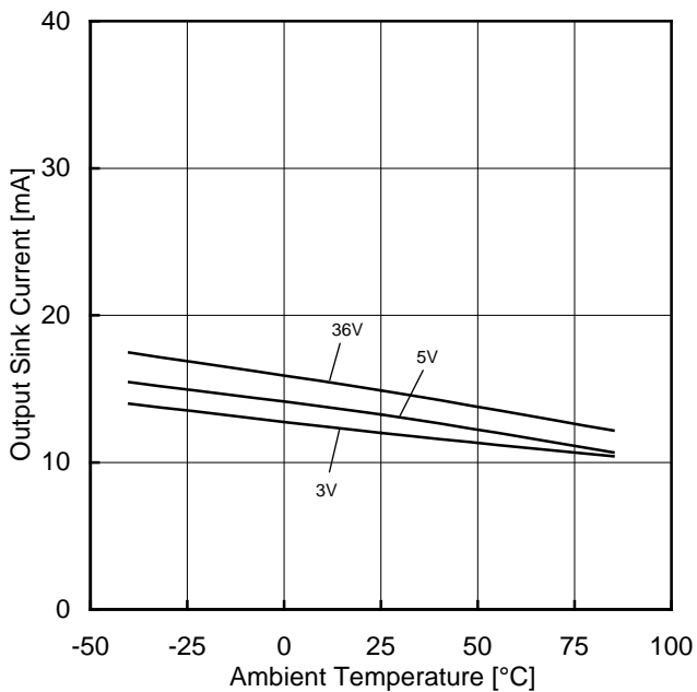
Figure 51. 出力シンク電流－温度特性 ( OUT=1.5V )
