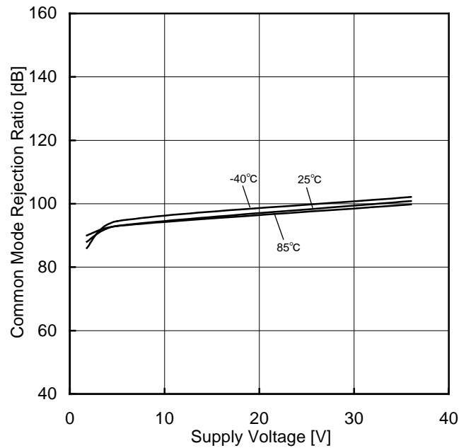
Figure 60. 同相信号除去比－電源電圧特性
