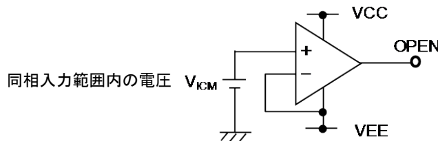
Figure 117. 未使用回路の処理例
