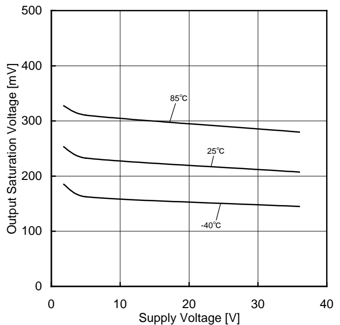
Figure 48. 出力飽和電圧—電源電圧特性 ( I_{SINK}=4mA )
