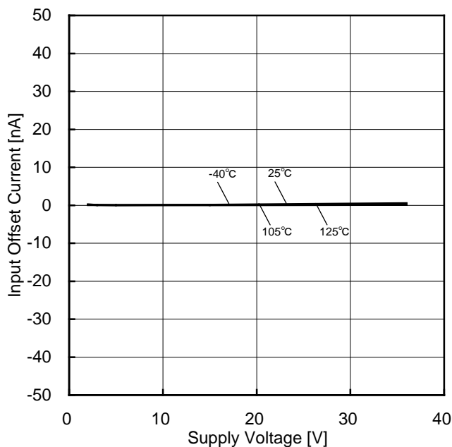
Figure 99. 入力オフセット電流-電源電圧特性
