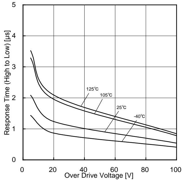
Figure 109. H→L 応答時間-オーバードライブ電圧特性 (VCC=5V, VRL=5V, RL=5.1kΩ)
