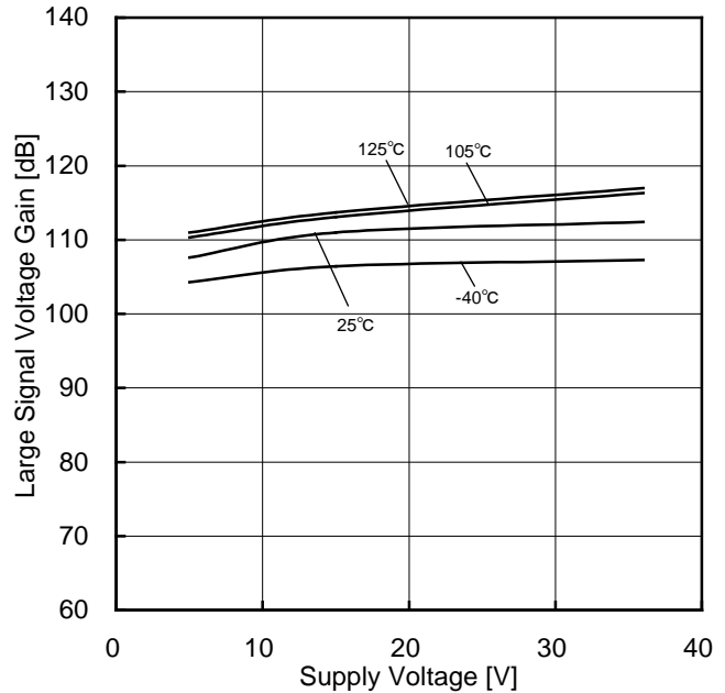
Figure 101. 大振幅電圧利得-電源電圧特性
