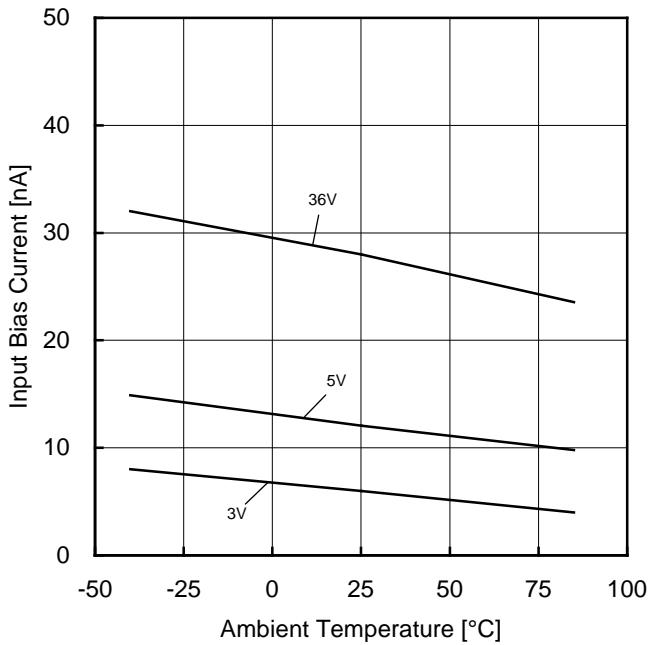
Figure 55. 入力バイアス電流-温度特性
