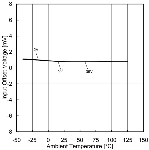
Figure 73. 入力オフセット電圧-温度特性
