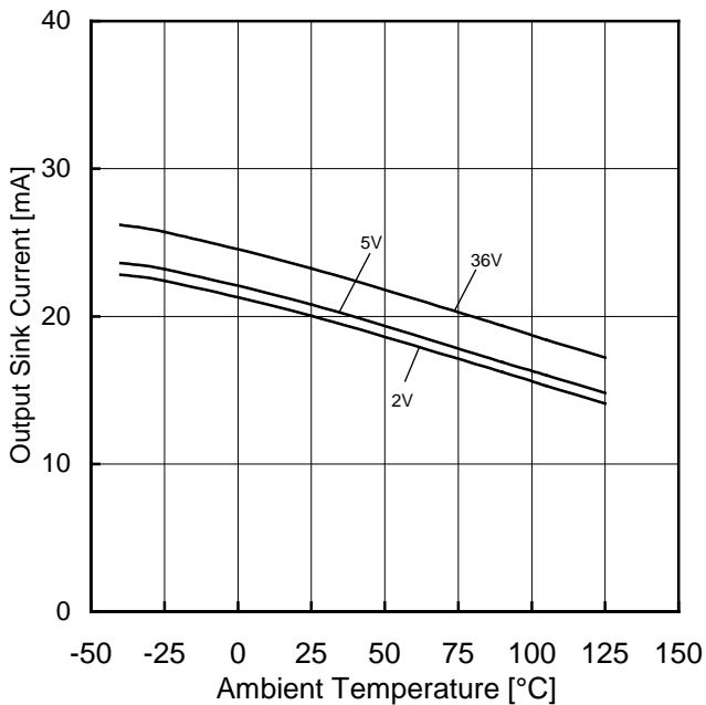
Figure 94. 出力シンク電流-温度特性 ( OUT=1.5V )
