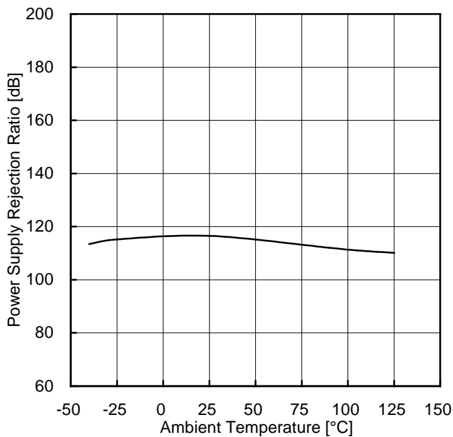
Figure 106. 電源電圧除去比-温度特性
