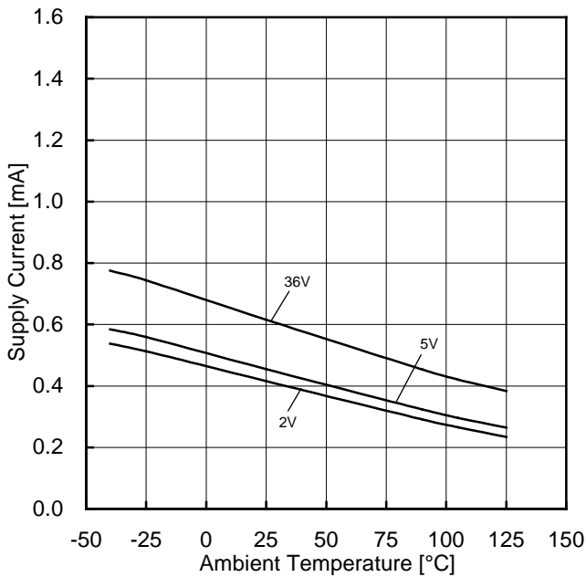
Figure 67. 回路電流-温度特性
