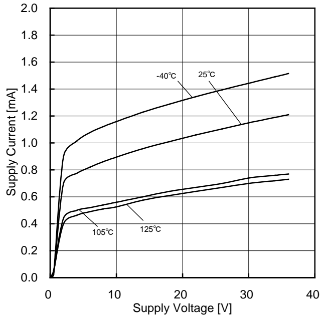
Figure 89. 回路電流-電源電圧特性
