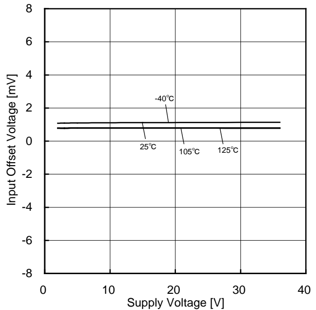
Figure 95. 入力オフセット電圧-電源電圧特性
