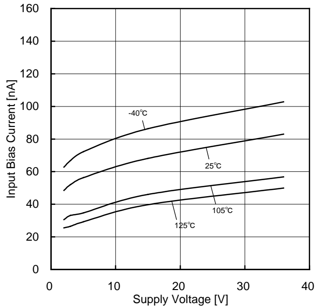
Figure 74. 入力バイアス電流-電源電圧特性
