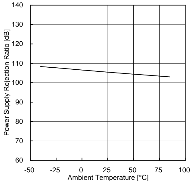
Figure 62. 電源電圧除去比-温度特性
