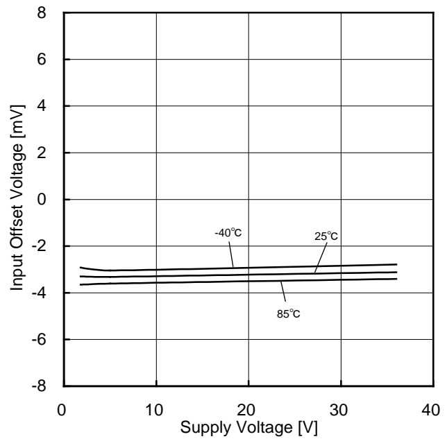
Figure 52. 入力オフセット電圧－電源電圧特性
