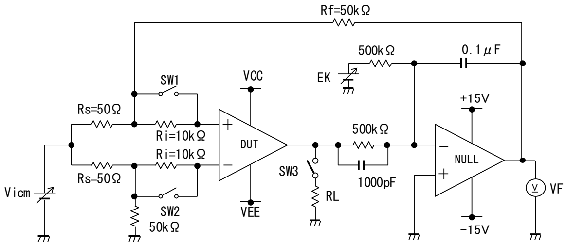
Figure 111. 測定回路 1 (1 チャンネルのみ)
