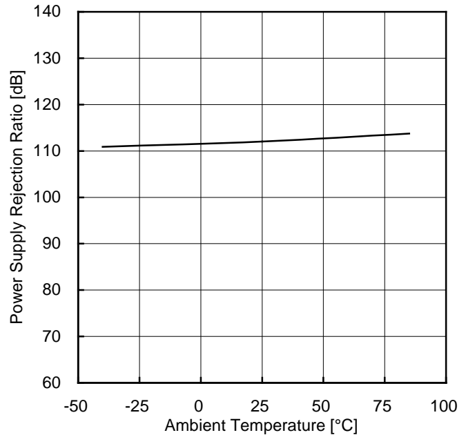
Figure 42. 電源電圧除去比-温度特性
