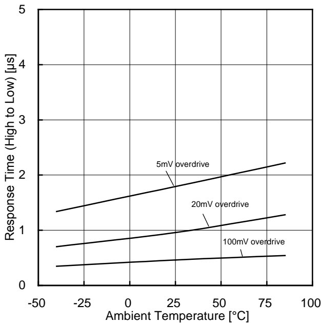
Figure 24. H→L 応答時間-温度特性 (VCC=5L=5V, RL=5.1kΩ)
