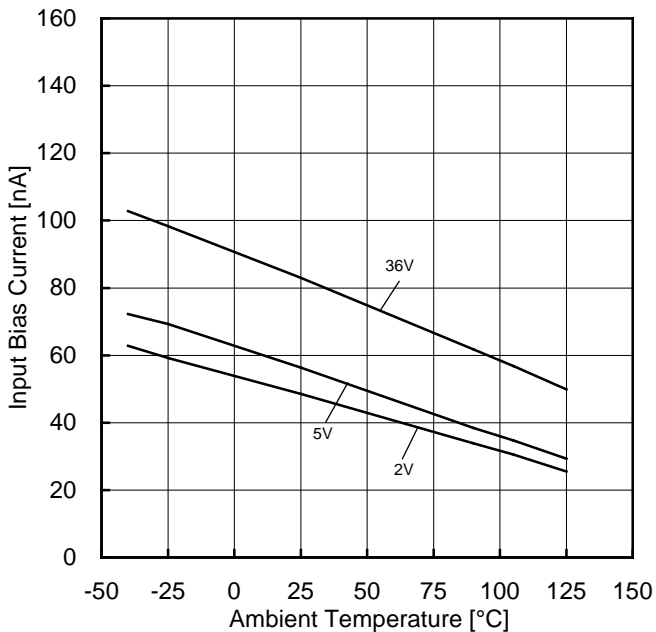
Figure 75. 入力バイアス電流-温度特性
