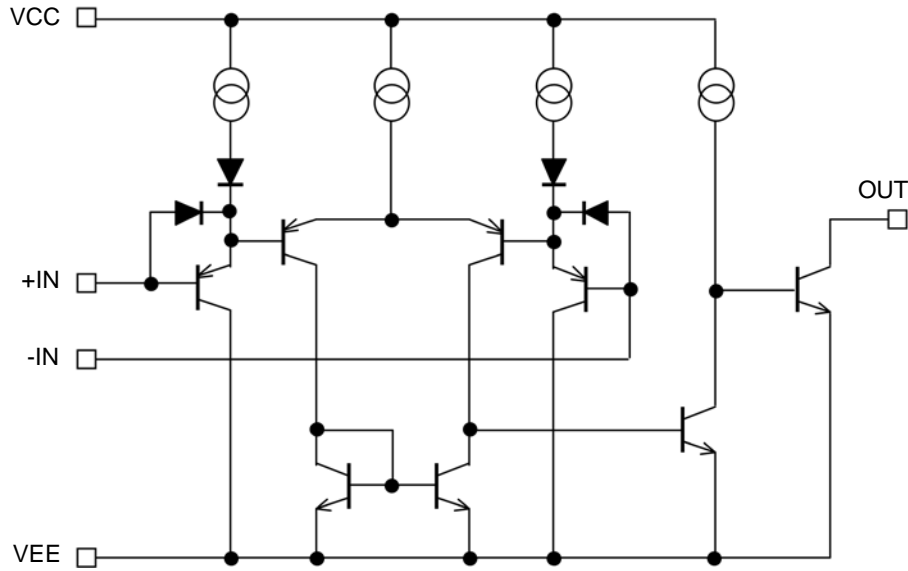
Figure 1. 内部等価回路図 (1チャンネルのみ)
