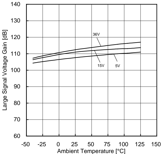
Figure 102. 大振幅電圧利得-温度特性
