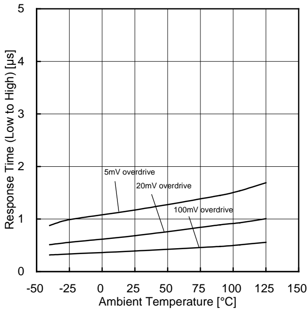
Figure 85. L→H 応答時間-温度特性 (VCC=5V, VRL=5V, RL=5.1kΩ)
