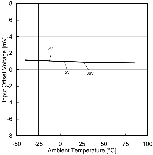
Figure 10. 入力オフセット電圧-温度特性
