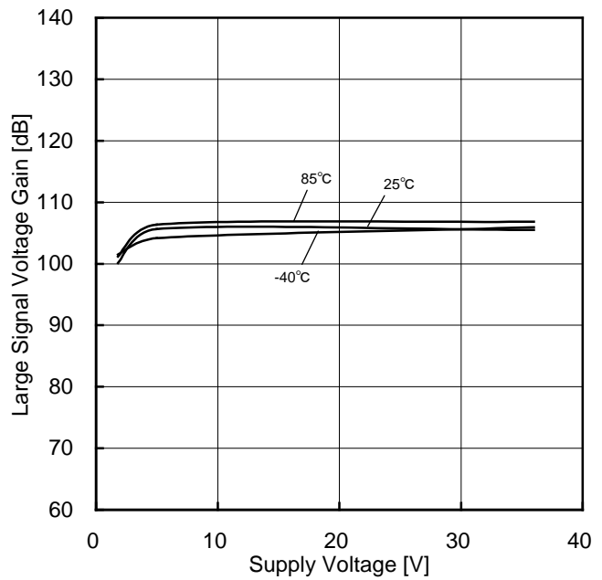
Figure 58. 大振幅電圧利得－電源電圧特性
