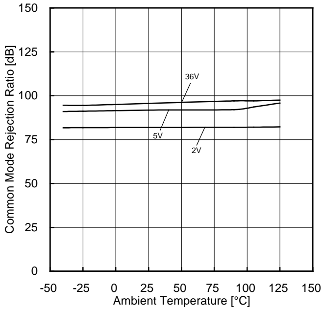
Figure 81. 同相信号除去比-温度特性
