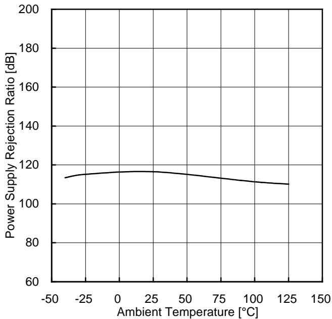
Figure 83. 電源電圧除去比-温度特性
