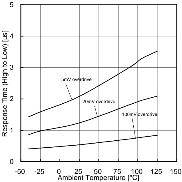
Figure 110. H→L 応答時間-温度特性 (VCC=5V, VRL=5V, RL=5.1kΩ)
