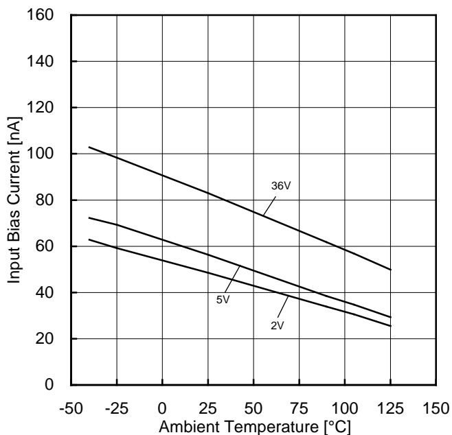
Figure 98. 入力バイアス電流-温度特性
