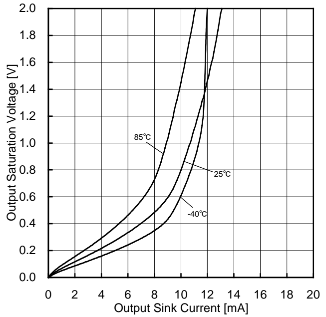
Figure 50. 出力飽和電圧－出力シンク電流 ( VCC=5V )
