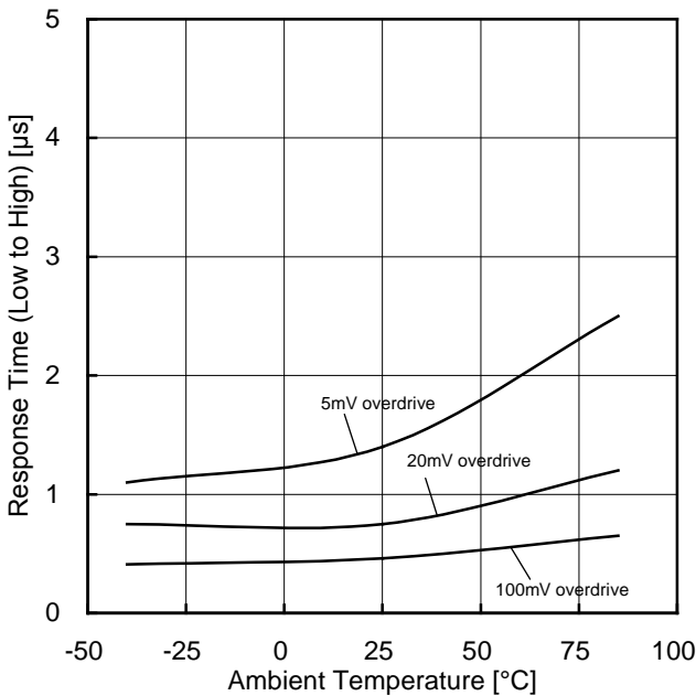
Figure 43. L→H 応答時間-温度特性 (VCC=5V, VRL=5V, RL=5.1kΩ)
