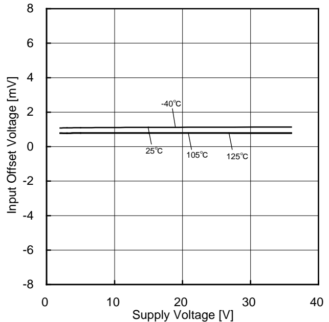
Figure 72. 入力オフセット電圧-電源電圧特性
