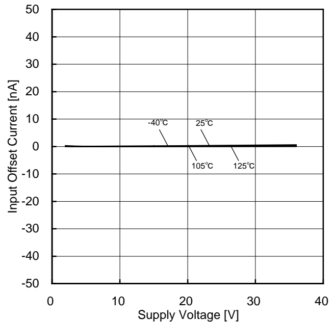
Figure 76. 入力オフセット電流-電源電圧特性
