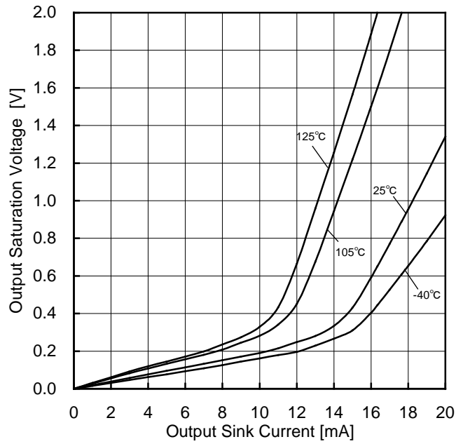
Figure 93. 出力飽和電圧-出力シンク電流特性 ( VCC=5V )
