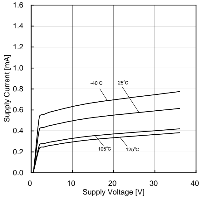
Figure 66. 回路電流-電源電圧特性
