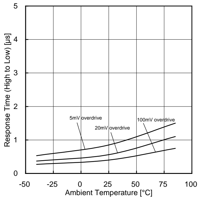
Figure 64. H→L 応答時間-温度特性 (VCC=5V, VRL=5V, RL=5.1kΩ)
