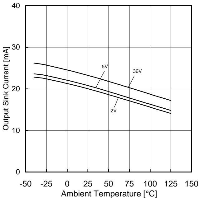
Figure 71. 出力シンク電流-温度特性 ( OUT=1.5V )
