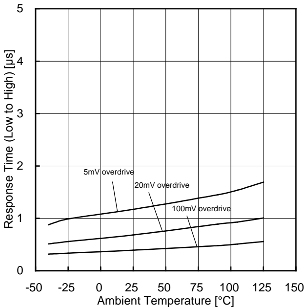
Figure 108. L→H 応答時間-温度特性 (VCC=5V, VRL=5V, RL=5.1kΩ)
