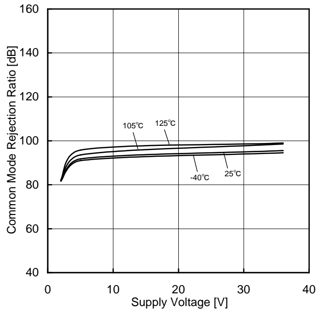
Figure 103. 同相信号除去比-電源電圧特性
