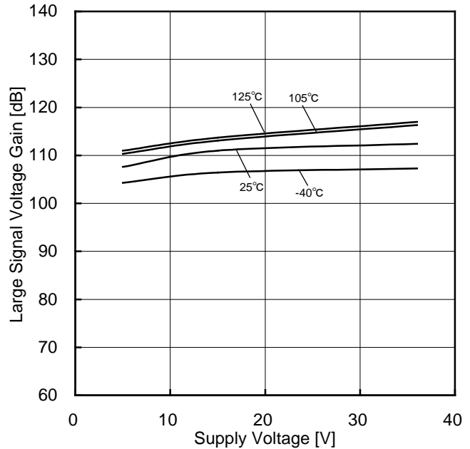
Figure 78. 大振幅電圧利得-電源電圧特性
