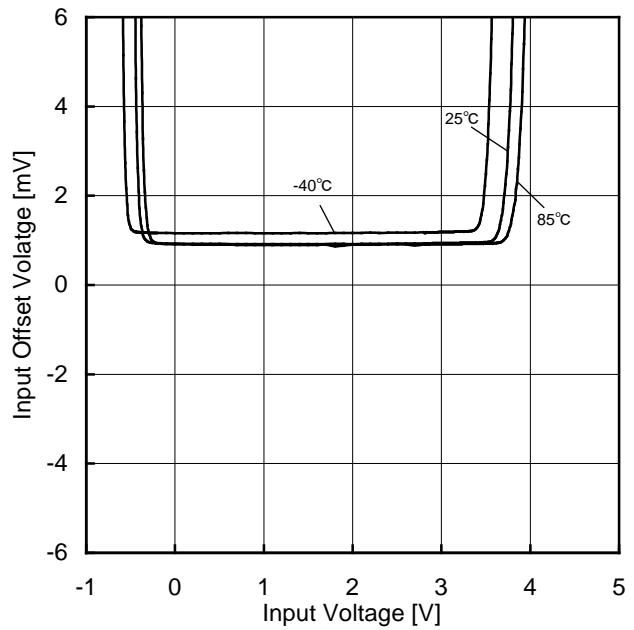
Figure 19. 入力オフセット-同相入力電圧範囲 (VCC=5V)
