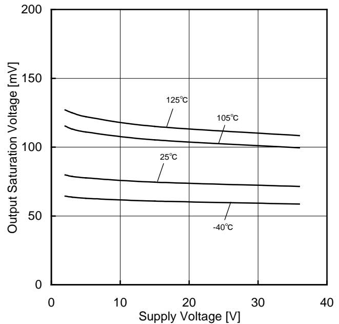
Figure 91. 出力飽和電圧-電源電圧特性 (I SINK =4mA)
