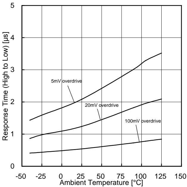
Figure 87. H→L 応答時間-温度特性 (VCC=5V, VRL=5V, RL=5.1kΩ)
