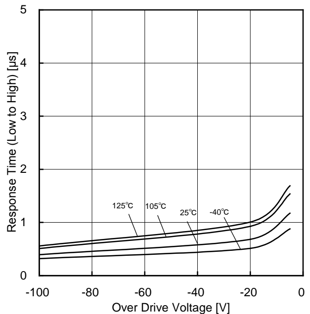
Figure 84. L→H 応答時間-オーバードライブ電圧特性 (VCC=5V, VRL=5V, RL=5.1kΩ)
