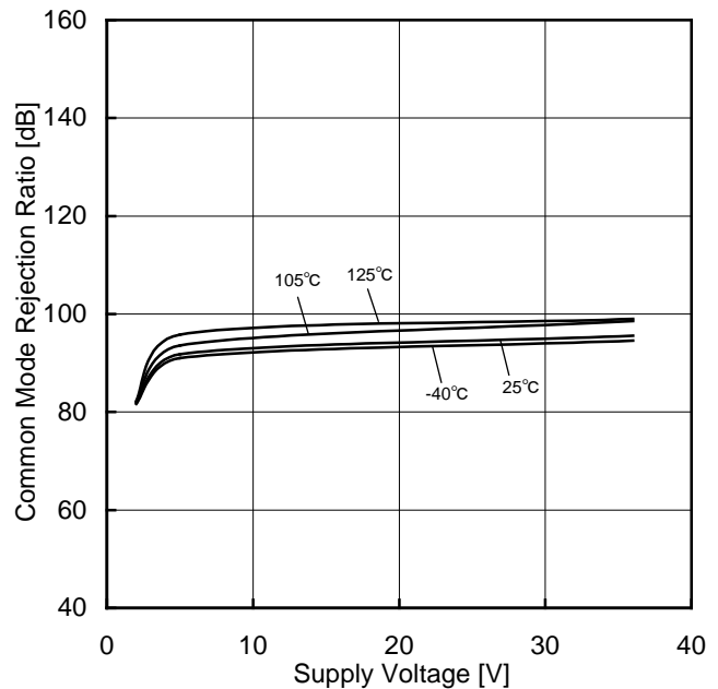
Figure 80. 同相信号除去比-電源電圧特性
