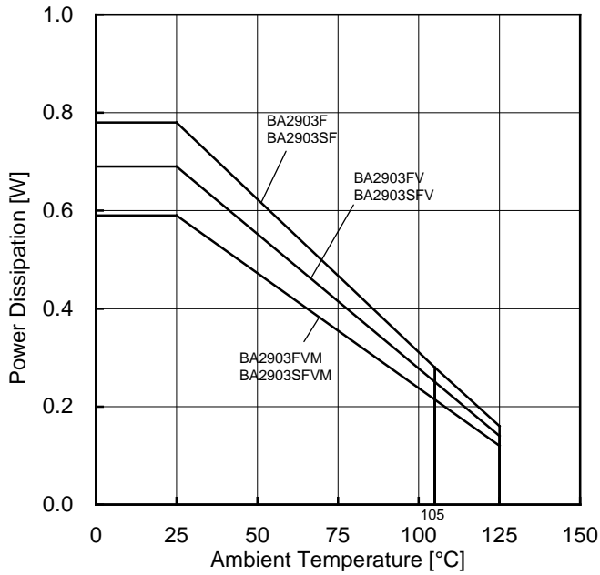
Figure 65. ディレーティングカーブ
