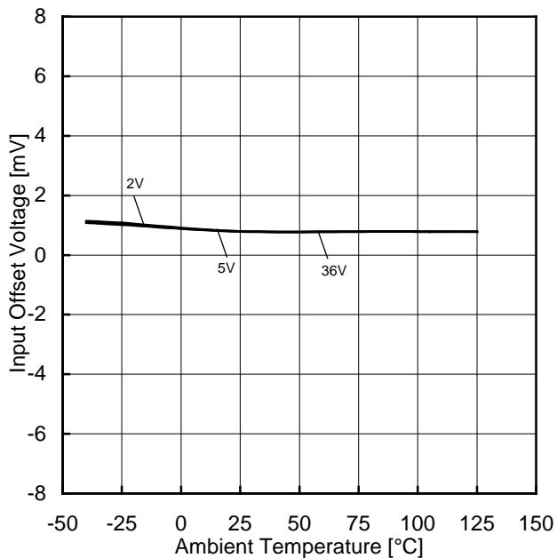
Figure 96. 入力オフセット電圧-温度特性
