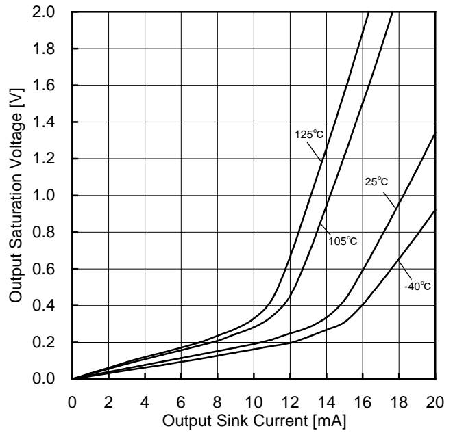
Figure 70. 出力飽和電圧-出力シンク電流特性 ( V_{CC}=5V )
