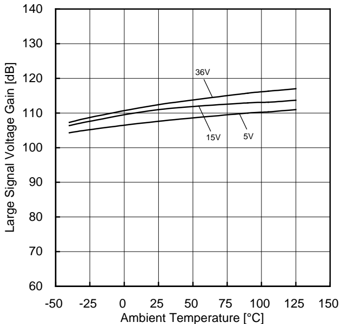
Figure 79. 大振幅電圧利得-温度特性
