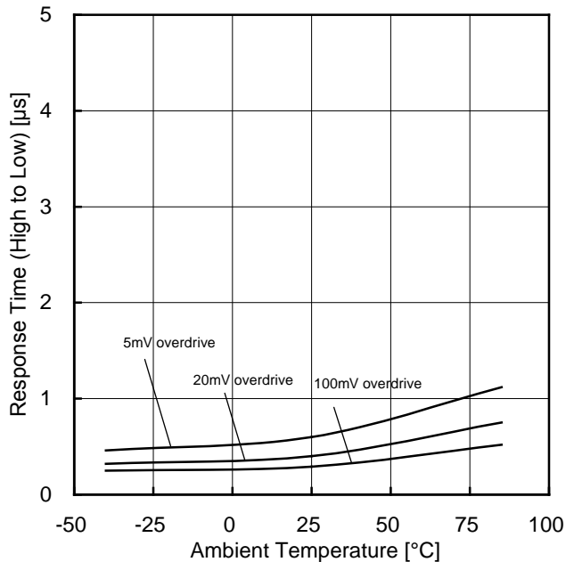
Figure 44. H→L 応答時間-温度特性 (VCC=5V, VRL=5V, RL=5.1kΩ)
