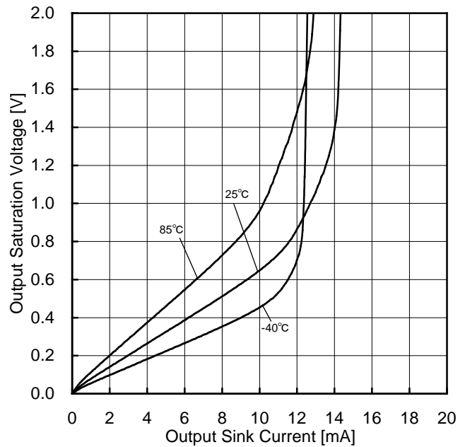
Figure 30. 出力飽和電圧－出力シンク電流特性 ( VCC=5V )
