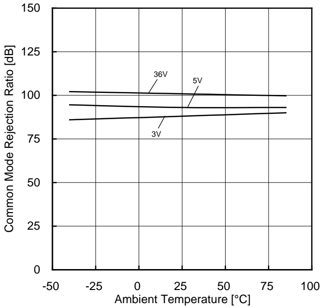
Figure 61. 同相信号除去比-温度特性
