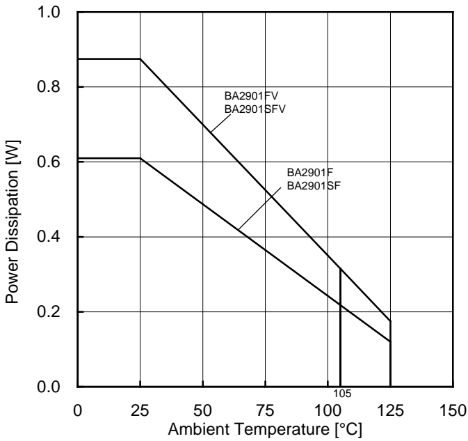
Figure 88. ディレーティングカーブ
