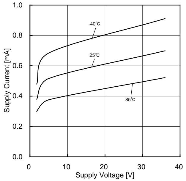
Figure 46. 回路電流—電源電圧特性
