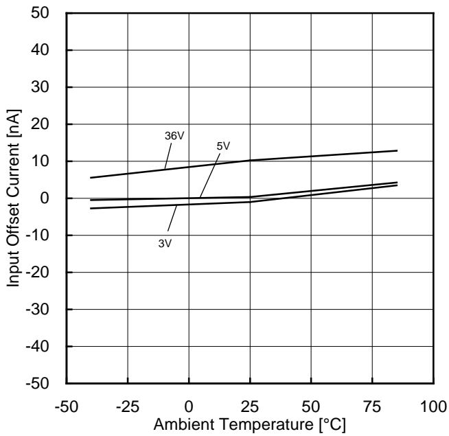
Figure 57. 入力オフセット電流－温度特性
