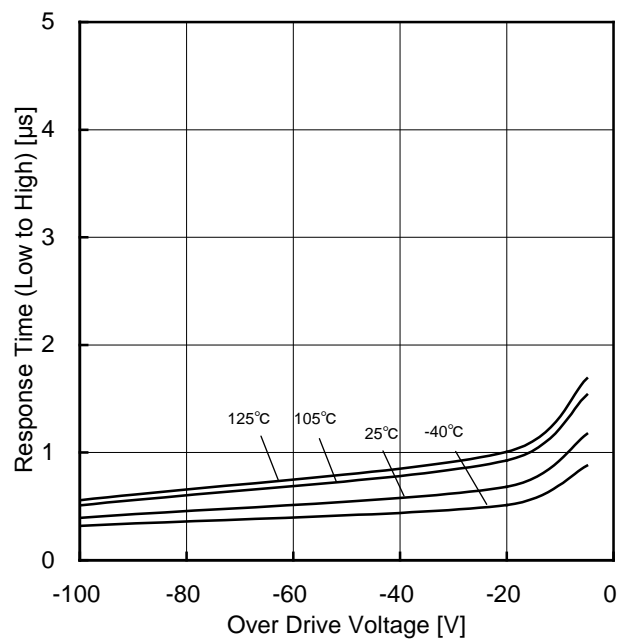
Figure 107. L→H 応答時間-オーバードライブ電圧特性 (VCC=5V, VRL=5V, RL=5.1kΩ)
