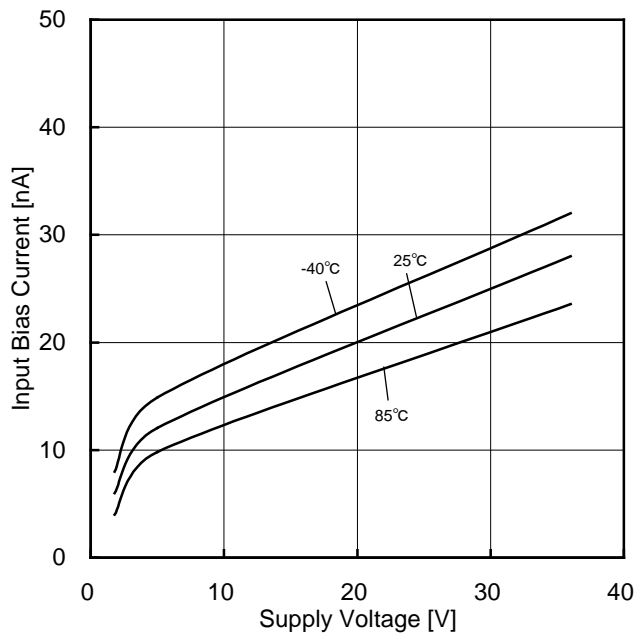
Figure 54. 入力バイアス電流-電源電圧特性
