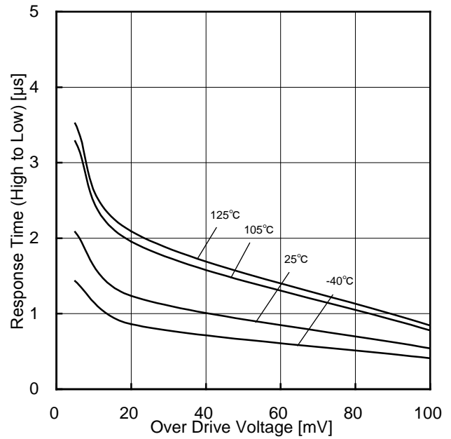
Figure 86. H→L 応答時間-オーバードライブ電圧特性 (VCC=5V, VRL=5V, RL=5.1kΩ)
