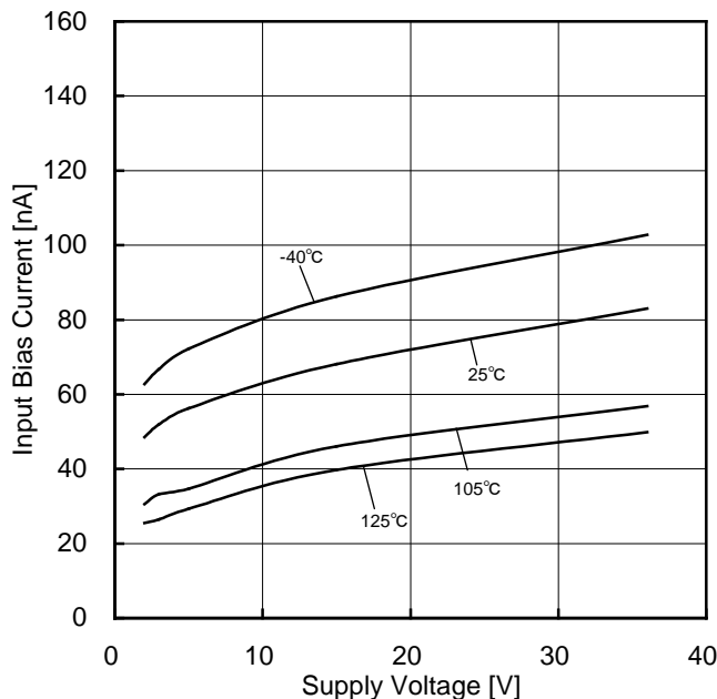
Figure 97. 入力バイアス電流-電源電圧特性
