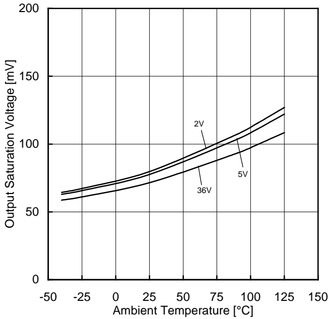
Figure 69. 出力飽和電圧-温度特性 ( I_{SINK}=4mA )
