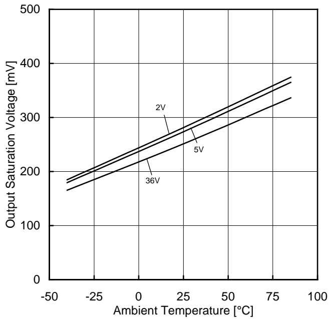
Figure 29. 出力飽和電圧－温度特性 ( I_{SINK}=4mA )
