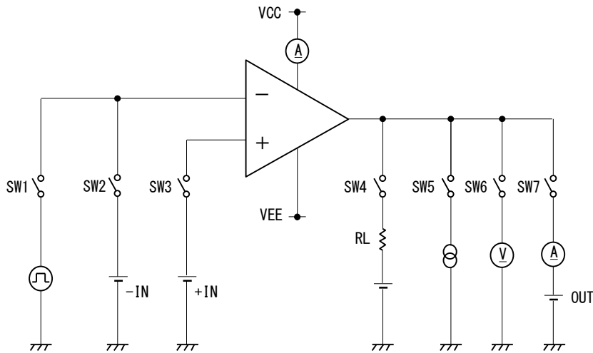
Figure 112. 測定回路 2 (片チャンネルのみ)
