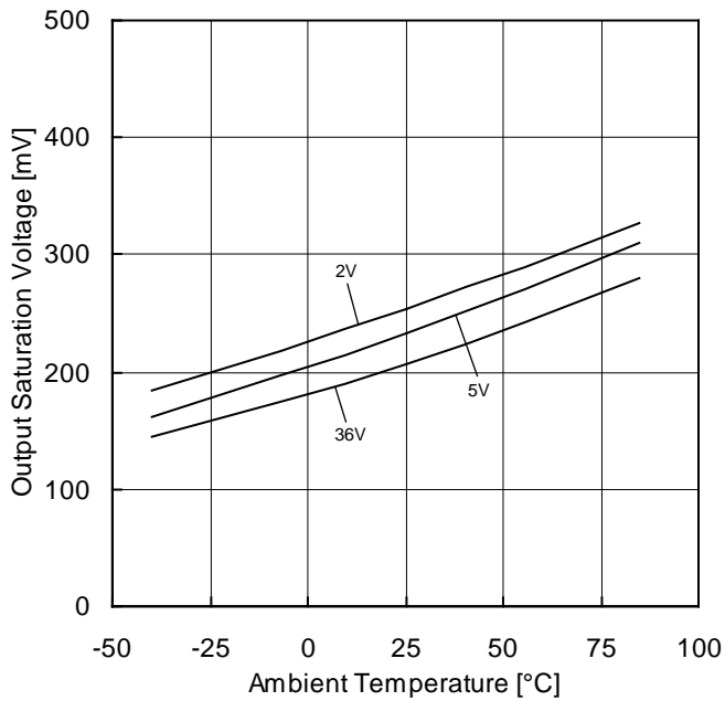
Figure 49. 出力飽和電圧－温度特性 ( I_{SINK}=4mA )
