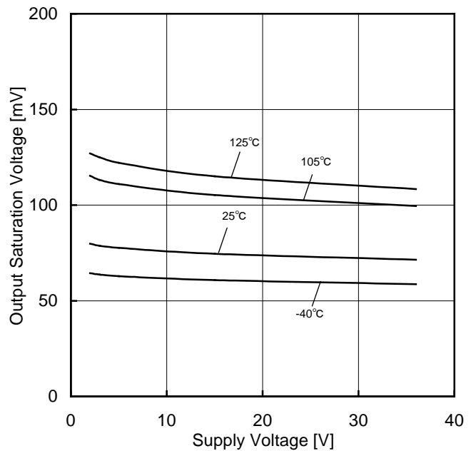
Figure 68. 出力飽和電圧-電源電圧特性 ( I_{SINK}=4mA )
