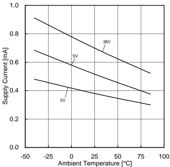
Figure 47. 回路電流—温度特性
