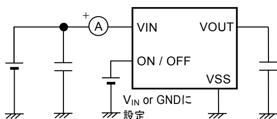
図12 測定回路2
