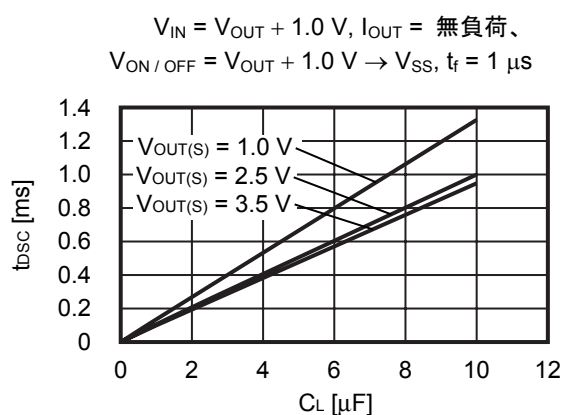
図22 S-1313シリーズA/Bタイプ (放電シャント機能あり)
