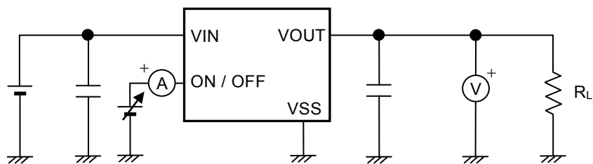
図14 測定回路4
