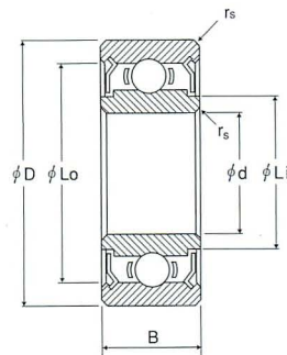
シールド付 Radial Shielded Ball Bearings
