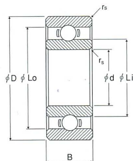
開放形 Radial Open Ball Bearings
