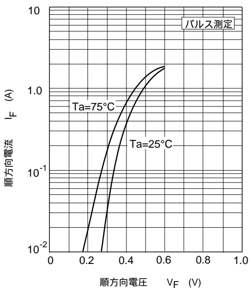
図1. 順方向特性
