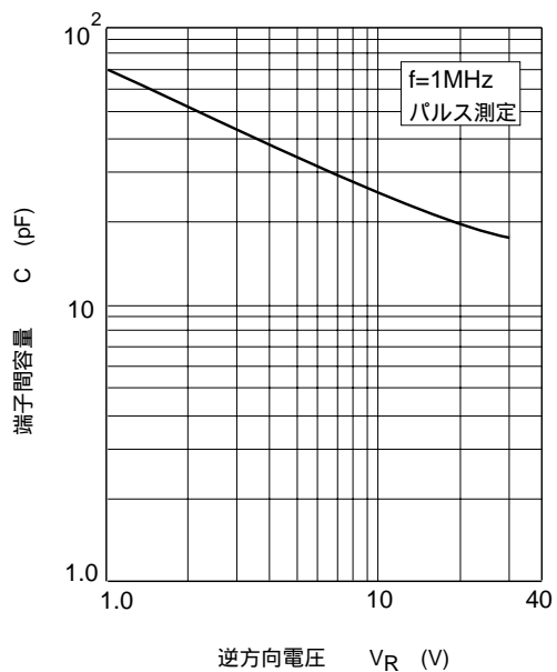
図3. 端子間容量 対 逆電圧特性
