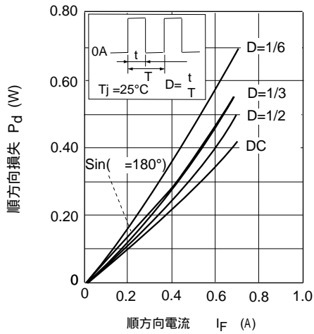
図4. 順方向損失 対 順電流特性
