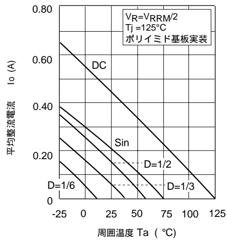
図7. 平均整流電流 対 周囲温度特性
