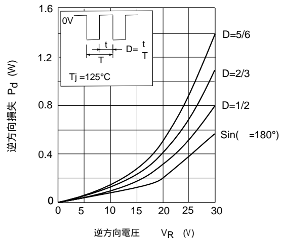
図5. 逆方向損失 対 逆電圧特性
