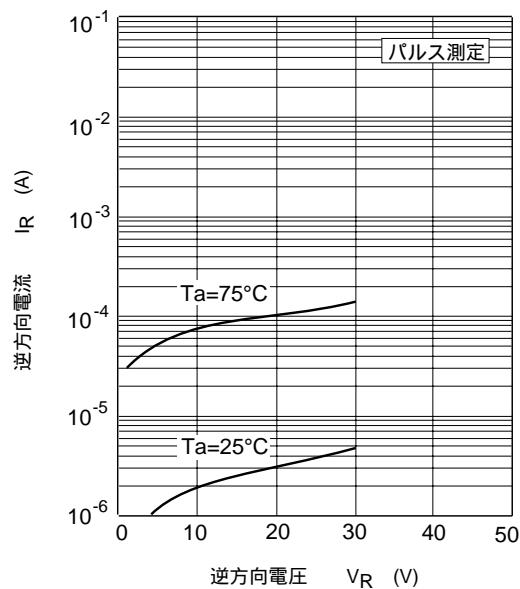
図2. 逆方向特性
