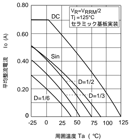
図6. 平均整流電流 対 周囲温度特性
