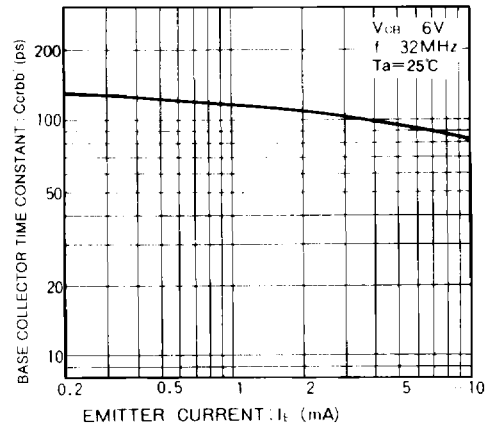
Fig.14 ベース・コレクタ時定数—エミッタ電流特性
