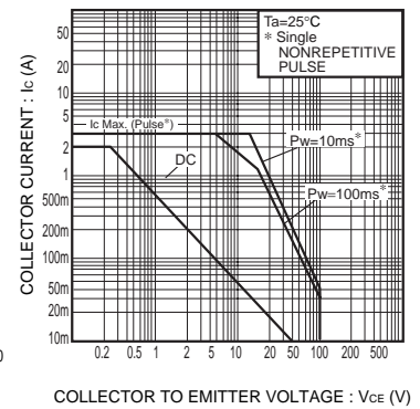
Fig.6 安全動作領域(A.S.O) (2SB1580)
