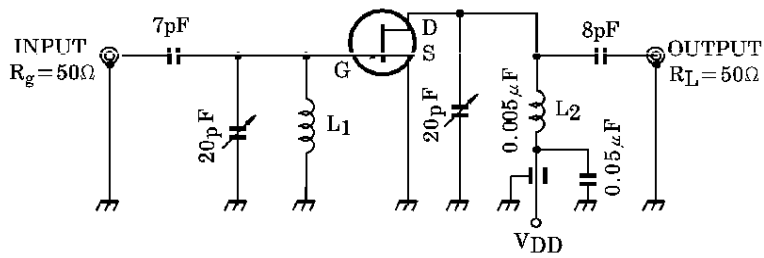
Fig. 100MHz G_{ps} NF TEST CIRCUIT
