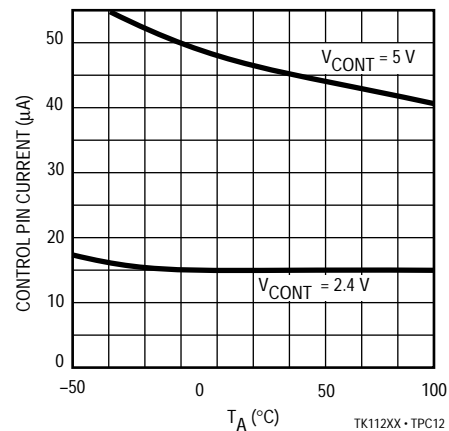
TK112XX · TPC12
