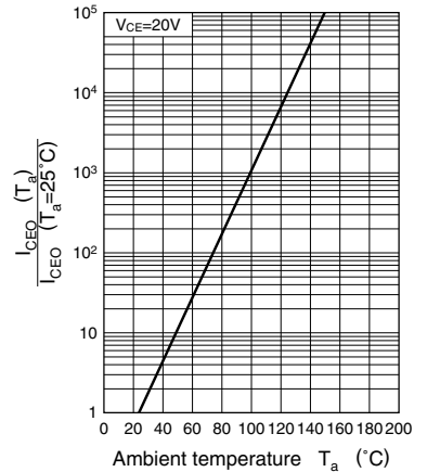
I_{CEO} - T_a
