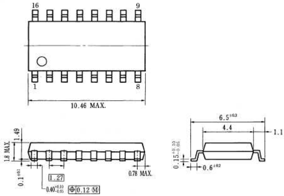
16ピン・プラスチック SOP (225 mil) 外形図(単位: mm)
