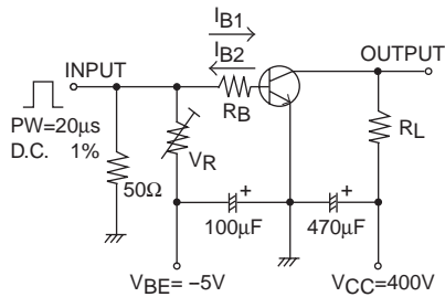
スイッチングタイム測定回路図
