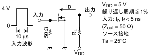
(a) 測定回路
