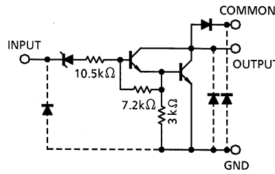
TD62002AP/AF
