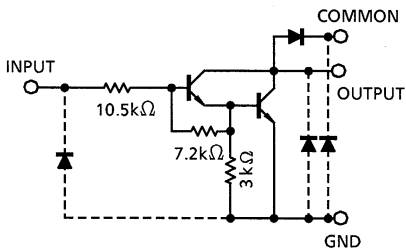
TD62004AP/AF
