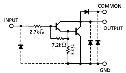
TD62003AP/AF
